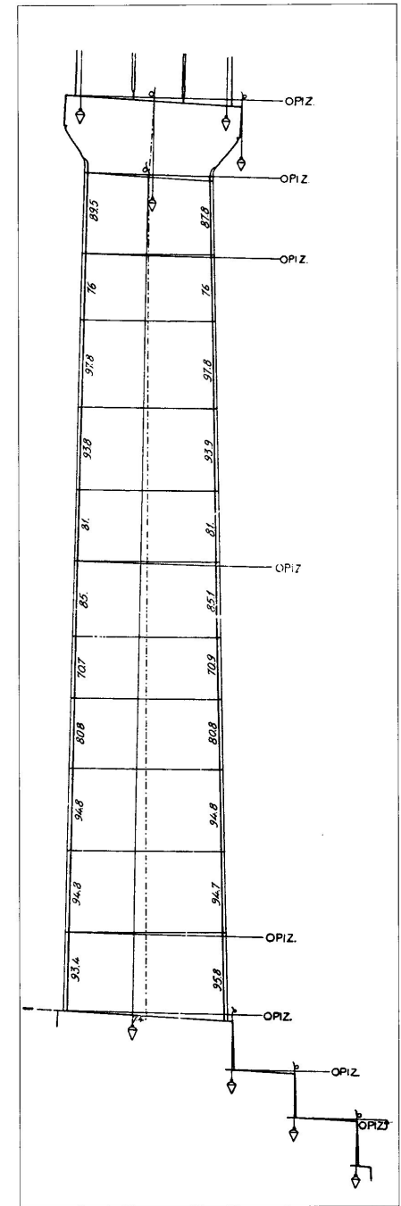
Fig. 271. Athènes, Parthénon. Schéma de l'inclinaison des colonnes et de la crépis. D'après Orlandos 1977, fig. 111.
